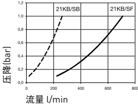
气体流量
