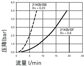
水流量
